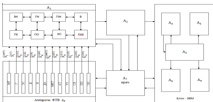
Рисунок 1. Блок – схема АЛДС.
