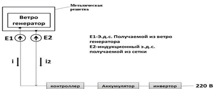
Рисунок 2. Ветро-энергосистема с магнитными лопастями.
