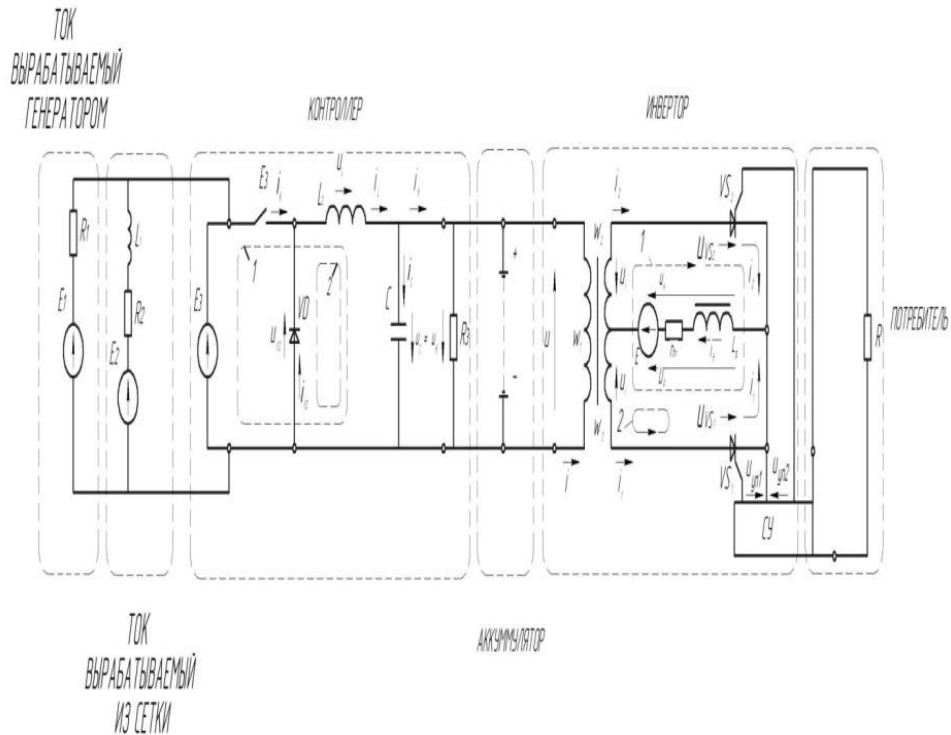
Рисунок 3. Электрическая схема замещения ВЭУ с магнитными лопастями.
