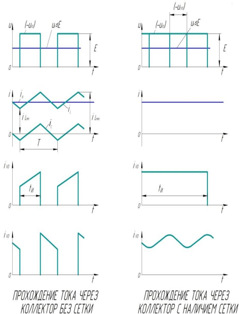
Рисунок 4-5. Вид тока на выходе контроллера.
